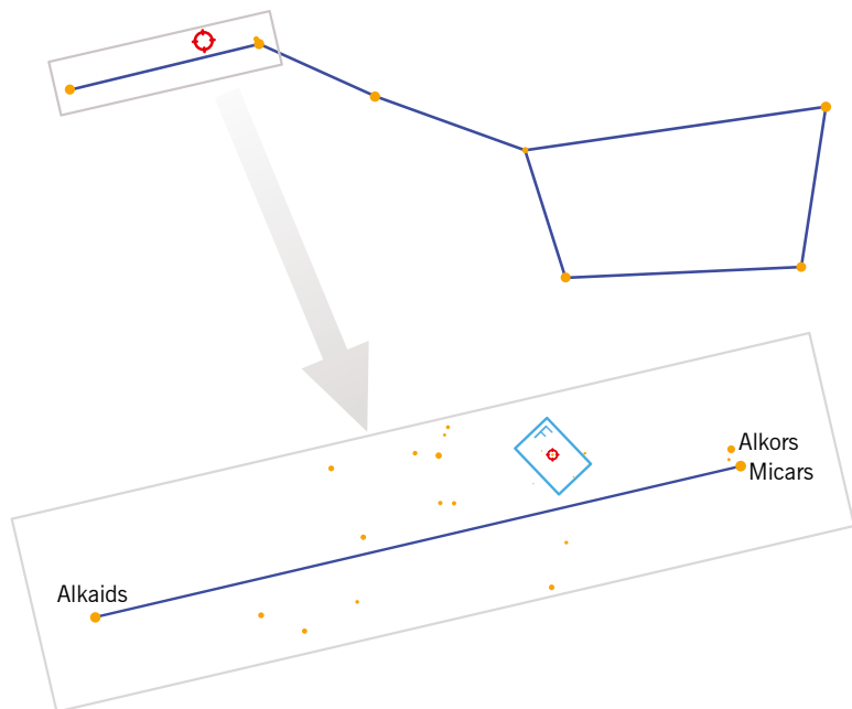
Shēma, kā atrast Liesmu Lielā Lāča zvaigznājā
