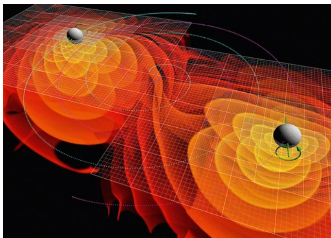
Divu melno caurumu saplūšanas simulācija
