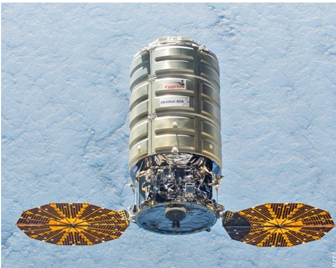
Kosmosa kuģis Cygnus tuvojas Starptautiskajai kosmosa stacijai
