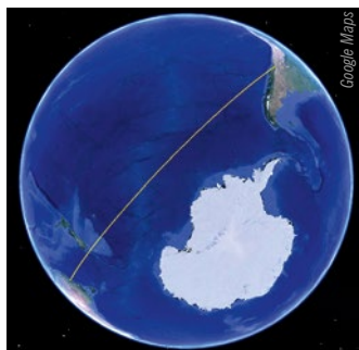
Lidojuma maršruts no Austrālijas uz Čīli apaļās un plakanās Zemes gadījumā
