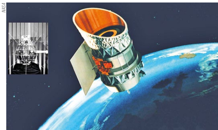
Satelīti Poppy VII-B un IRAS
