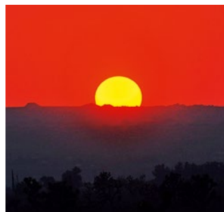
Saule noriet aiz horizonta, nevis virs horizonta, kā tam vajadzētu būt, ja Zeme būtu plakana
