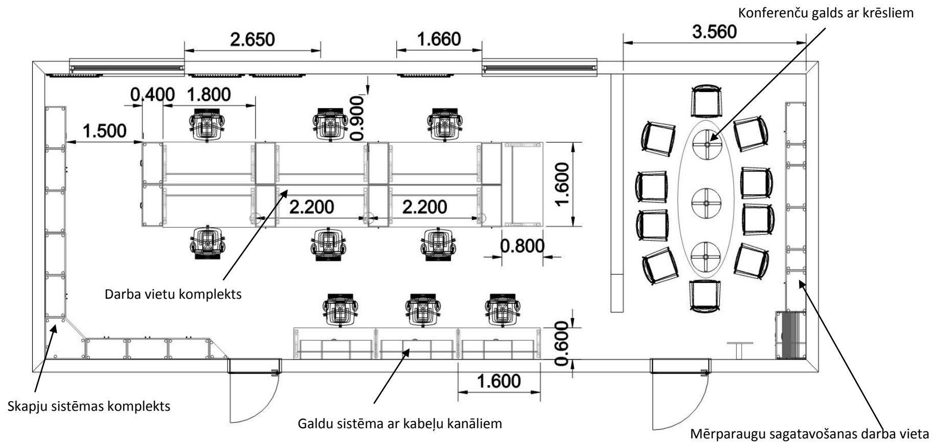
Telpu plāni ar mēbeļu izvietojumu tehniskās specifikācijas punktiem. 4.-8.
